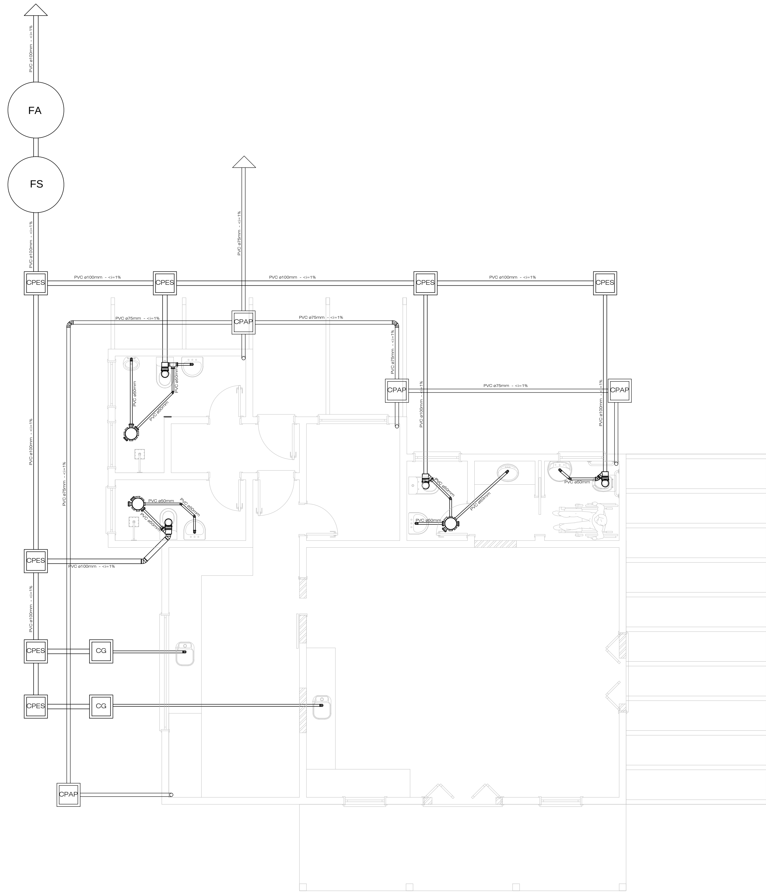
PLANTA BAIXA ESGOTO SANITÁRIO ESCALA: 1/50
